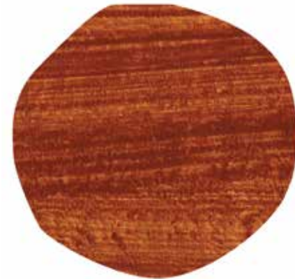
bruin | بني
